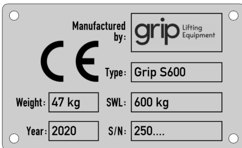
Bild 1: Typskylt
