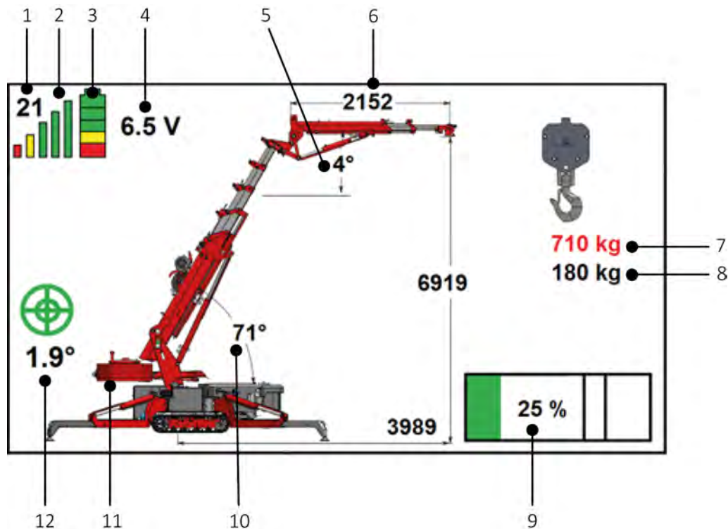
Figura 4.8 Display durante il sollevamento
