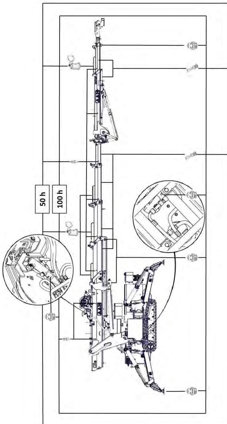
Figura 5.2 Schema di ingrassaggio
