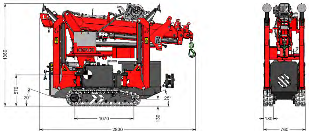
Figura 1.2 Vista frontale e laterale C4e con indicazione del baricentro
