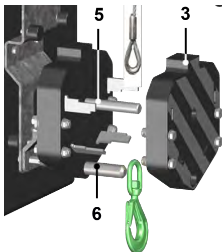
Figur 4.15 Fissaggio della fune e del gancio di sollevamento al bozzello
