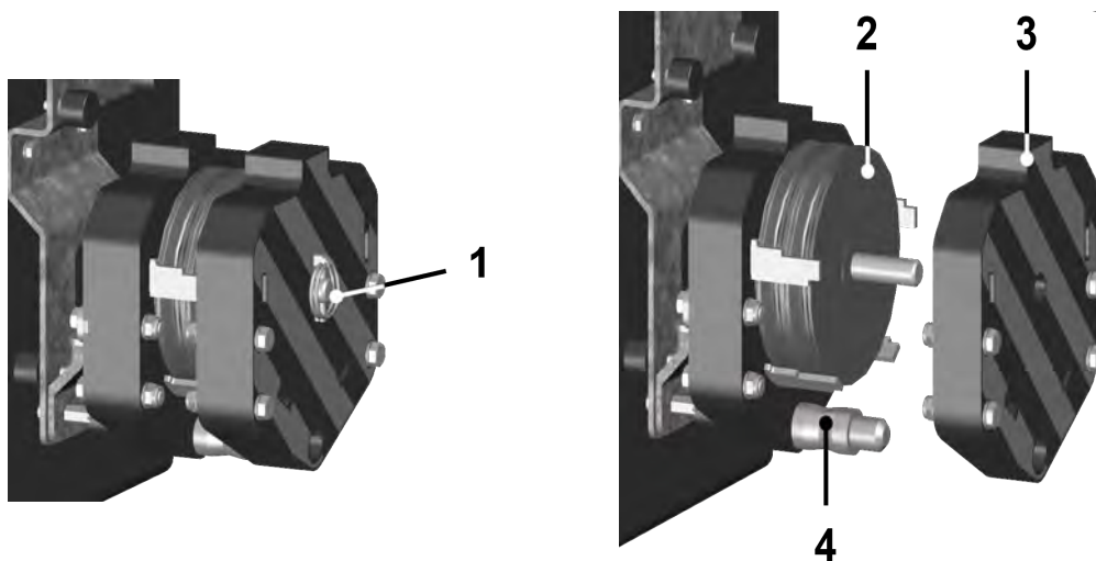
Figur 4.14 Rimuovere il bozzello
