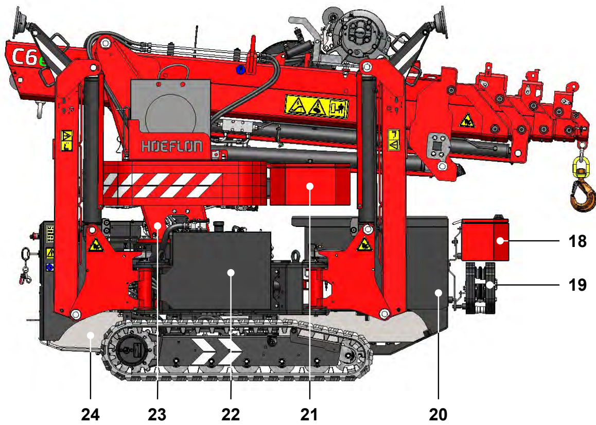
Figur 2.2 Vista lato destro C6e
