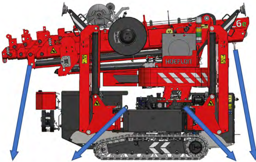
Figura 7.3 Immobilizzazione della gru
