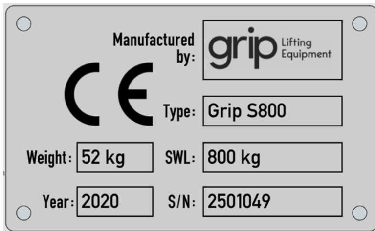
Ilustracja 1: Tabliczka znamionowa
